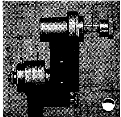
Bild 31 Spulenarmverlängerung a Raststift c Buchse b Filmspulenechse d Friktion e Rändelschraube
