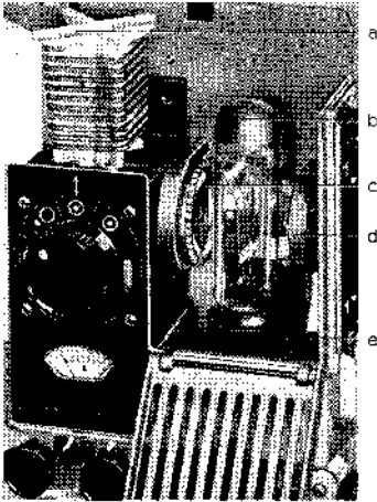
Bild 12 Blick ins Lampenhaus Schutzkappe abgenommen
