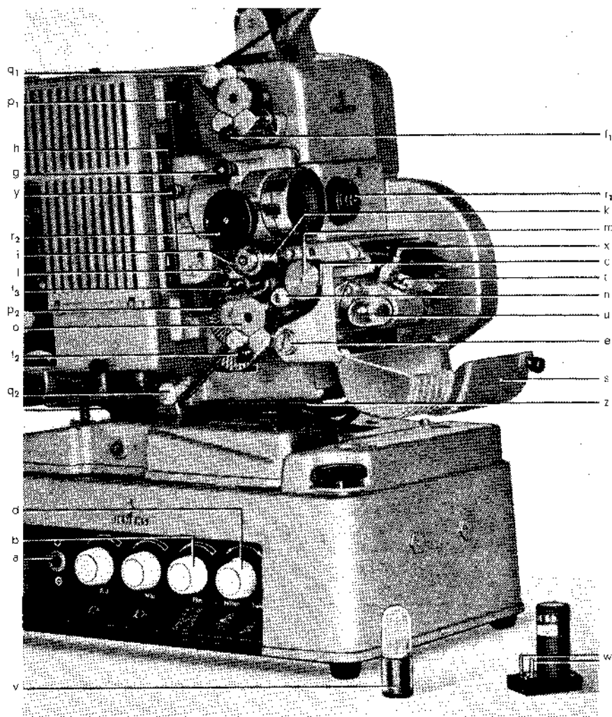
Bild 16 Projektor mit Lichtgerät und Verstärker
